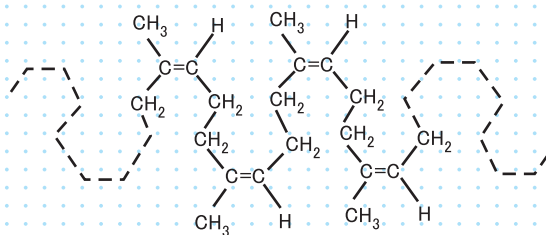
天然ゴムを作る高分子の構造
